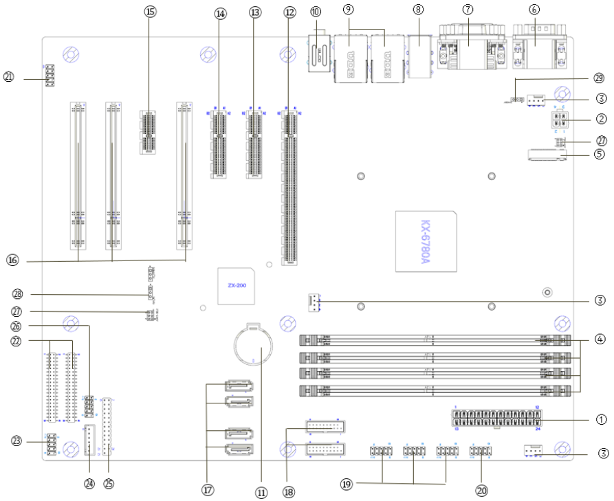
IZ28-A 接口位置图
